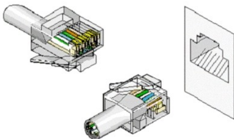
Рисунок 4-1. Разъем RJ-45
