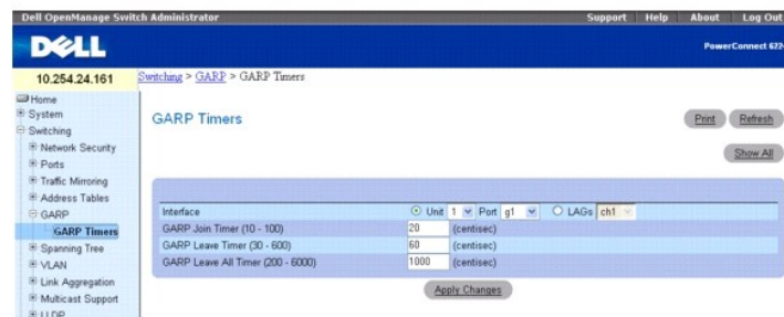
Рис. 7-33. Таймеры GARP
