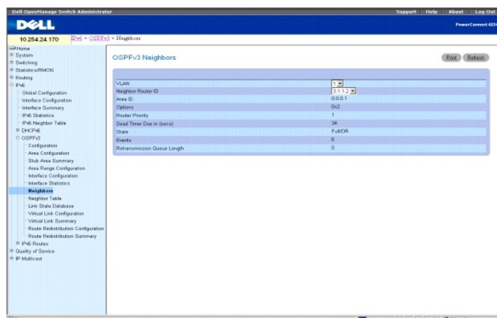
Рисунок 10-25. Соседи OSPFv3
